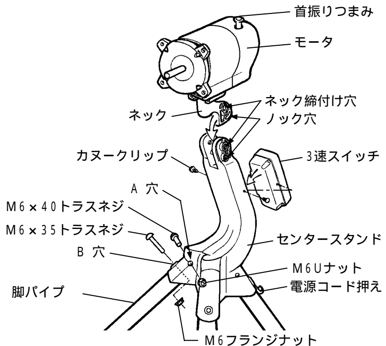
図示 ネックとセンタースタンドの固定
