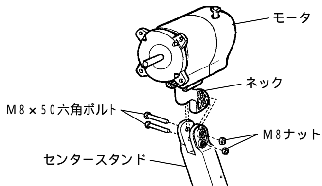
図示 ネックとセンタースタンドの固定
