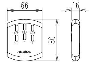
⑧リモコン 拡大図
