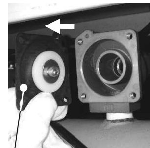
⑦ダイヤフラム弁
