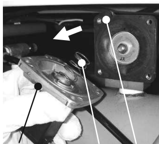
⑥ケーシング バネ ピン
