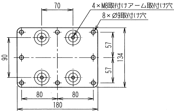
取付脚穴寸法
