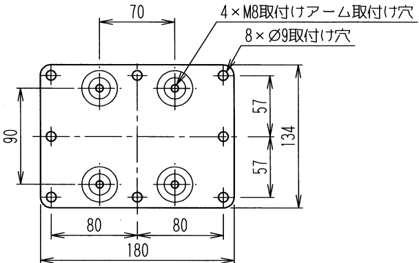
取付脚穴寸法
