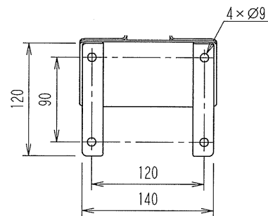
脚取付板穴寸法
