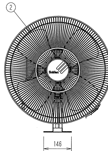
取付脚穴寸法
