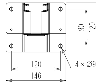
取付脚穴寸法
