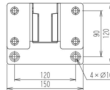
取付脚穴寸法
