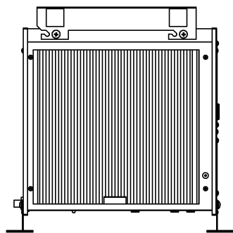
A矢視図
