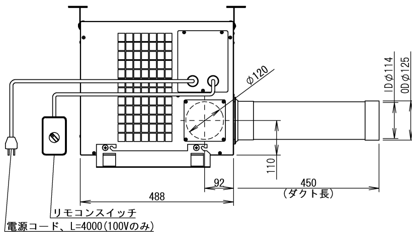
A矢視図
