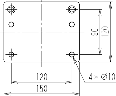
A 矢視図 (取付脚穴寸法)
